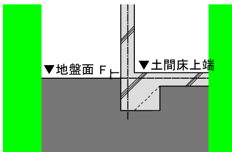
図1 土間床上端が地盤面と同じか高い場合の土間床上端と地盤面の高さの差
