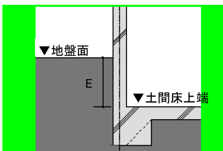
図2 土間床上端が地盤面より低い場合の土間床上端と地盤面の高さの差
