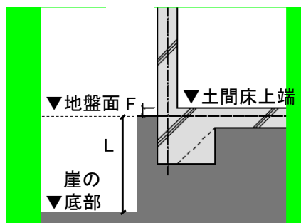
図3 土間床上端と崖の底部の差が1m 以上の場合
