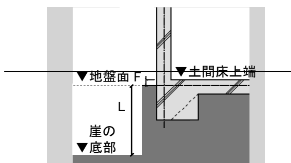
図3 土間床上端と崖の底部の差が1m以上の場合
