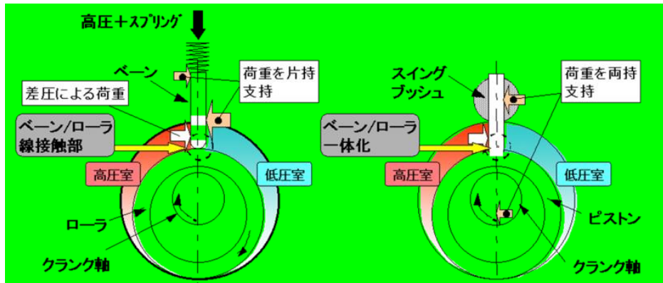
図 D.1 ロータリ式コンプレッサーの構造
