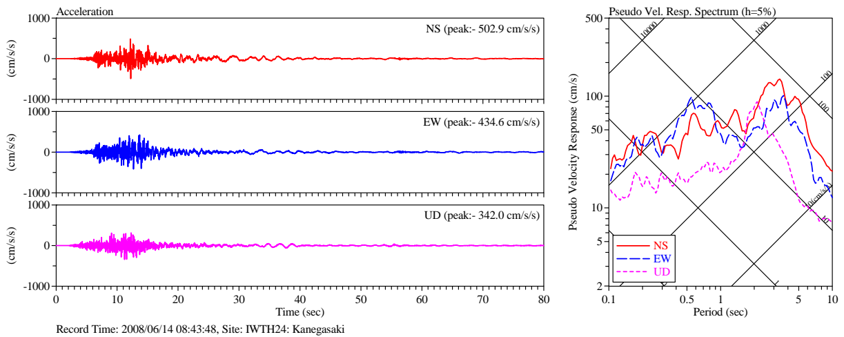
図-3.12 KiK-net 金ヶ崎 (IWITH24)の加速度記録と5%擬似速度応答スペクトル
