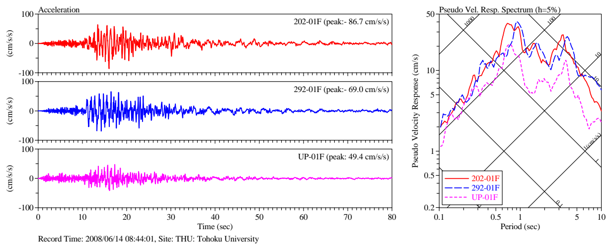
図-3.18 東北大学建設系建物 01F の加速度記録と 5%擬似速度応答スペクトル
