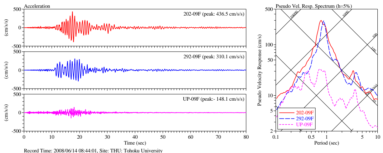
図-3.19 東北大学建設系建物 09F の加速度記録と 5%擬似速度応答スペクトル
