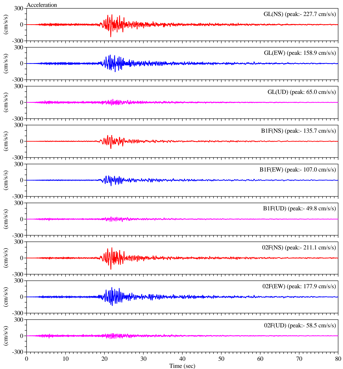
図-3.33 栗原文化会館地表(GL)、地下1階(B1F)及び2階(02F)の加速度記録。それぞれX成分(建物長辺方向)、Y成分(建物短辺方向)、Z成分(上下方向)の順で並ぶ
