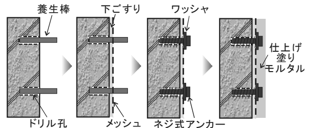
図 2 耐久性と防耐火性を両立させた補修工法の概要
