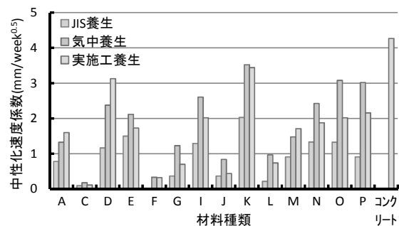
図 3 補修工法に使用する材料の促進中性化試験結果
