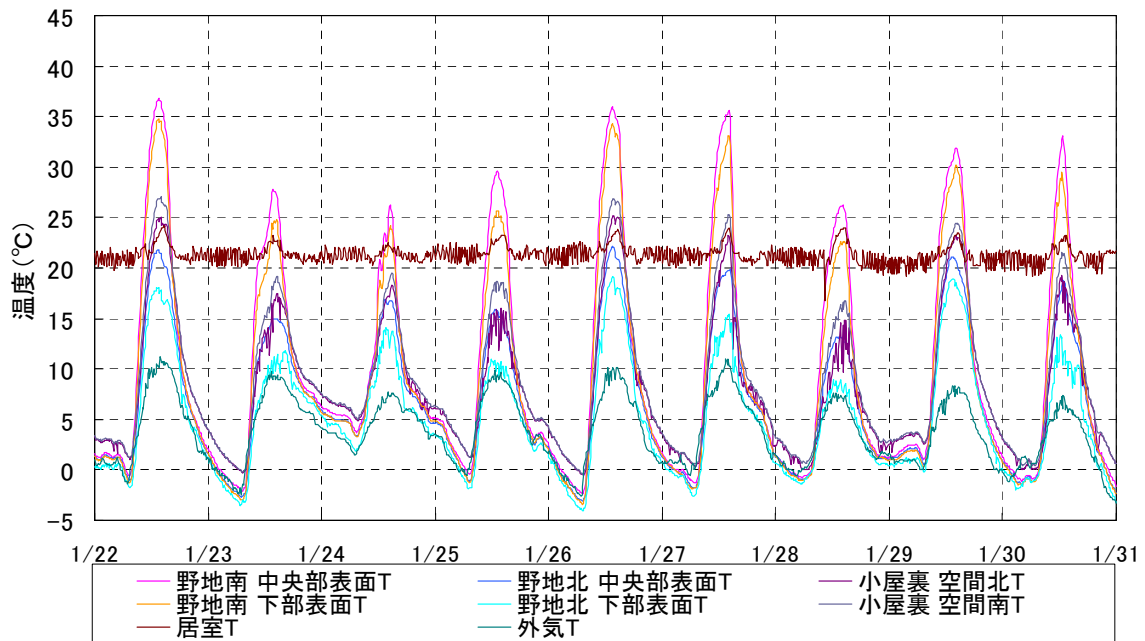
図 2.4.14 温度変動グラフ (Case10-4:1/22~1/30)
