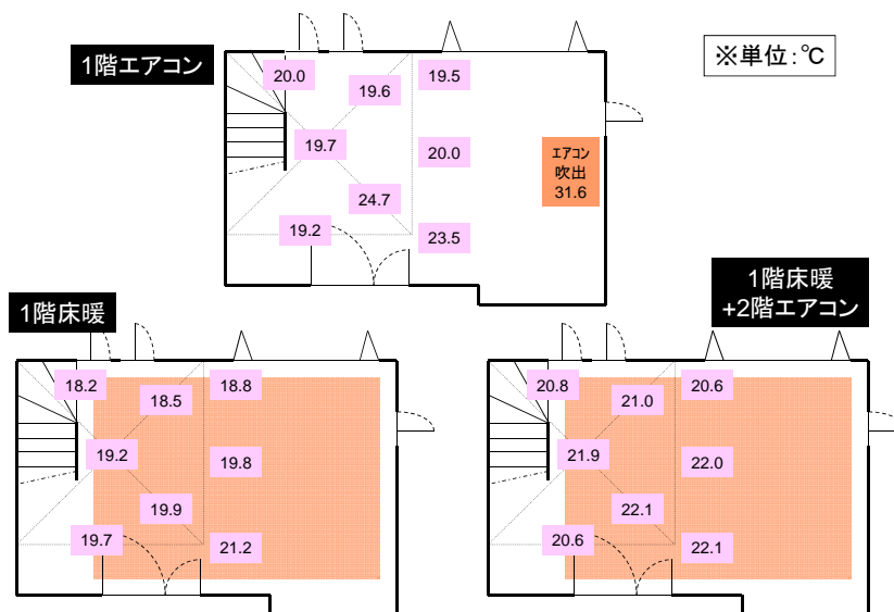
図 2.3.4 測定時の床付近温度分布
