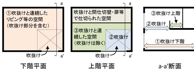
図 2.3.18 吹抜け及び吹抜けと連続した空間の床面積の定義
