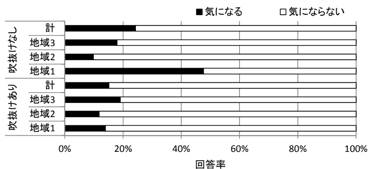
図 2.3.30 吹抜けの有無とまぶしさ
