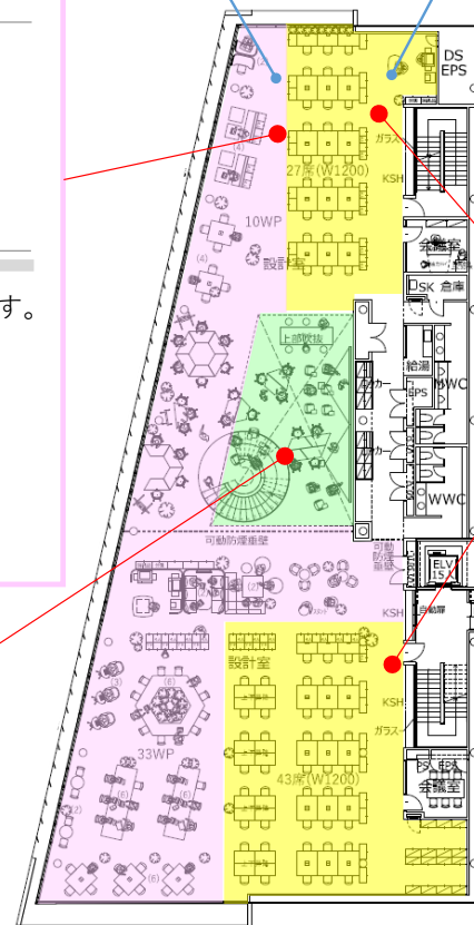
2階平面図
