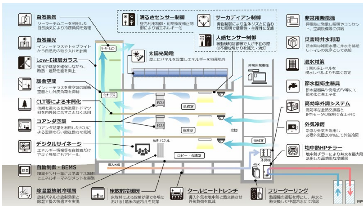
環境断面図
