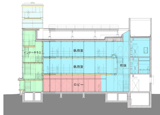
東西断面図
