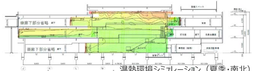
温熱環境シミュレーション (夏季・南北)
