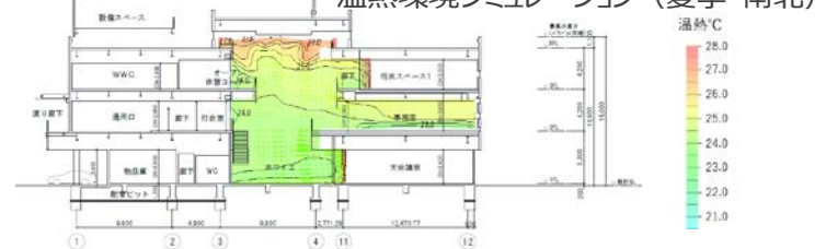
温熱環境シミュレーション (夏季・東西)
